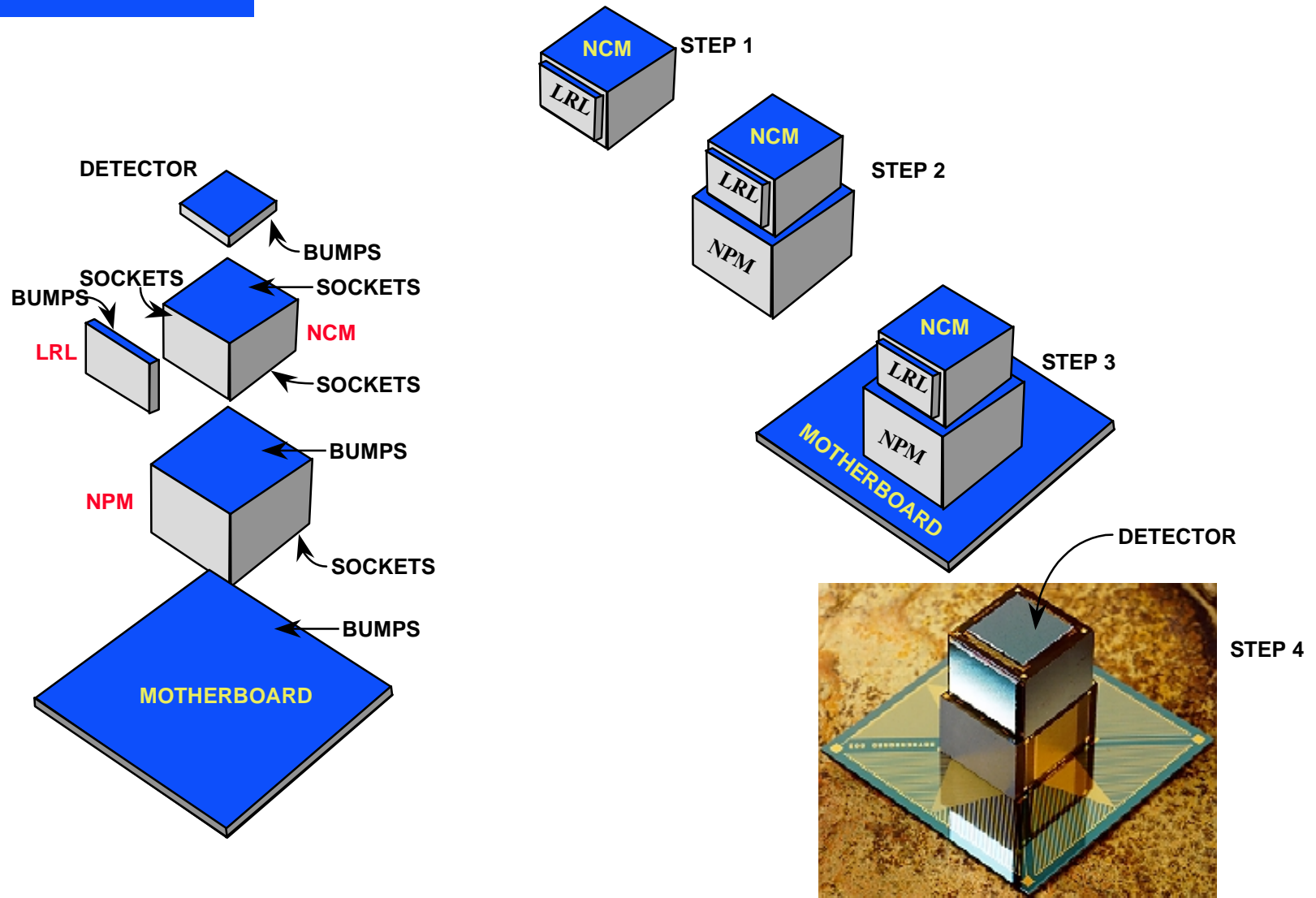
1 Tera-Op Processor
